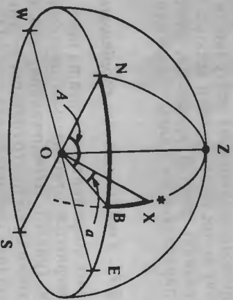
Рис. 5. Горизонтальные координаты.
