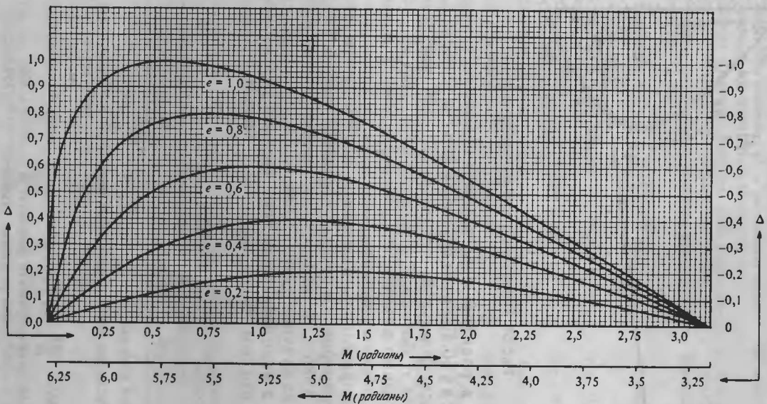
Рис. 28. График уравнения Кеплера. Левая шкала и верхняя шкала M предназначены для M между 0 и 3,14. Правая шкала и нижняя шкала M — для M между 3,14 и 6,28.
