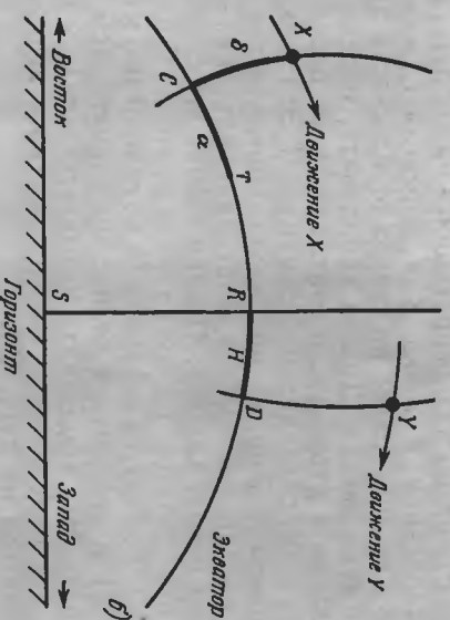
Рис. 6. Экваториальные координаты: а — на небесной сфере; б — при наблюдении с Земли.
