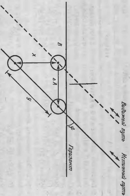
Рис 11 Истинное и видимое положения небесного тела при восходе и заходе.
