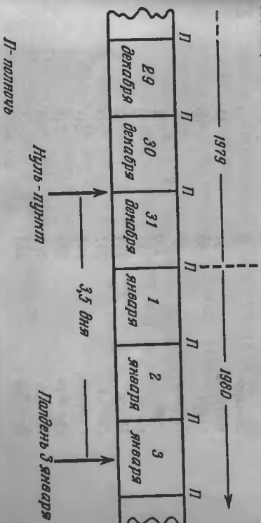
Рис. 1. Определение эпохи.
