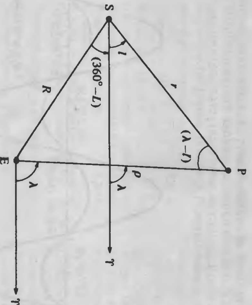
Рис 26 Определение расстояния до планеты
