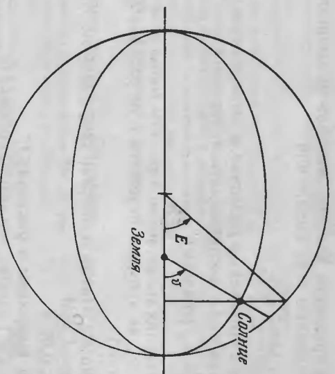
Рис. 19. Истинная аномалия и эксцентрическая аномалия.
