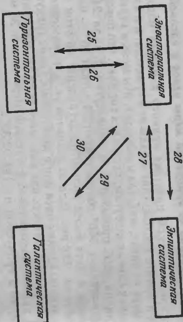
Рис. 9. Переход от одной системы координат к другой.
