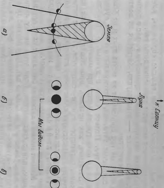
Рис. 38. а — лунное затмение; б — полное солнечное затмение; в — кольцевое солнечное затмение.
