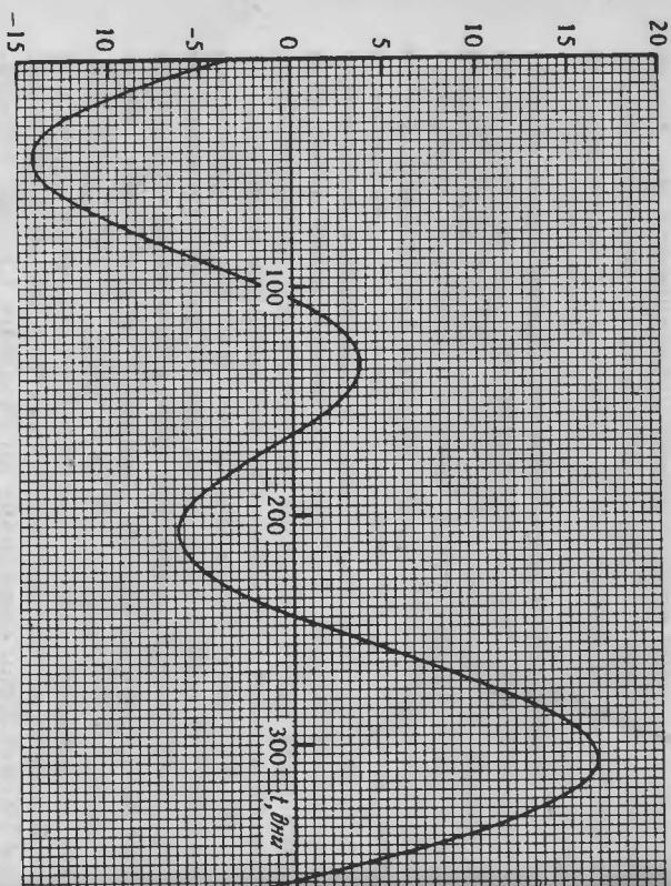
Рис. 20. Уравнение времени.
