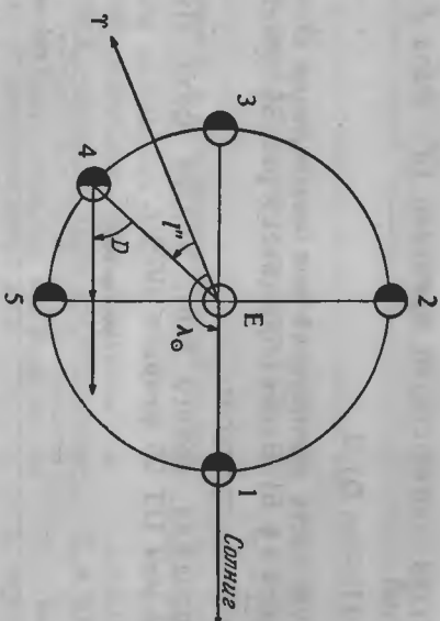
Рис. 35. Фазы Луны.
