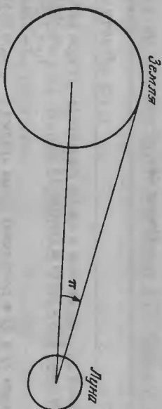
Рис. 36. Параллакс Луны.
