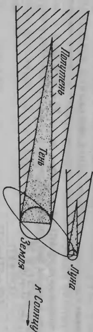
Рис. 37. Тени, отбрасываемые Луной и Землей.
