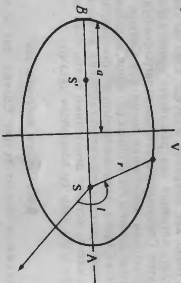
Рис. 17. Эллиптическая орбита.
