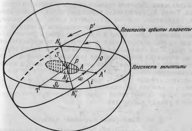
Рис. 21 Орбита планеты.
