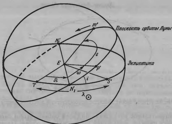
Рис. 33. Определение элементов орбиты Луны.
