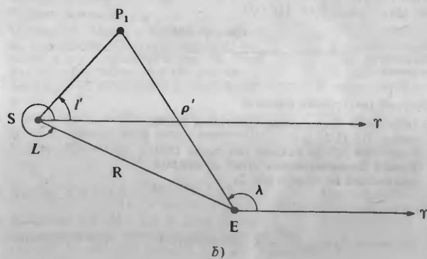
Рис. 23. Геометрия относительно плоскости эклиптики. а — внешняя планета; б — внутренняя планета.
