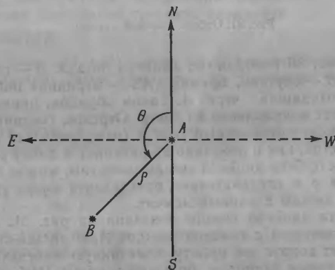
Рис. 30. Двойная звезда, наблюдаемая с Земли.
