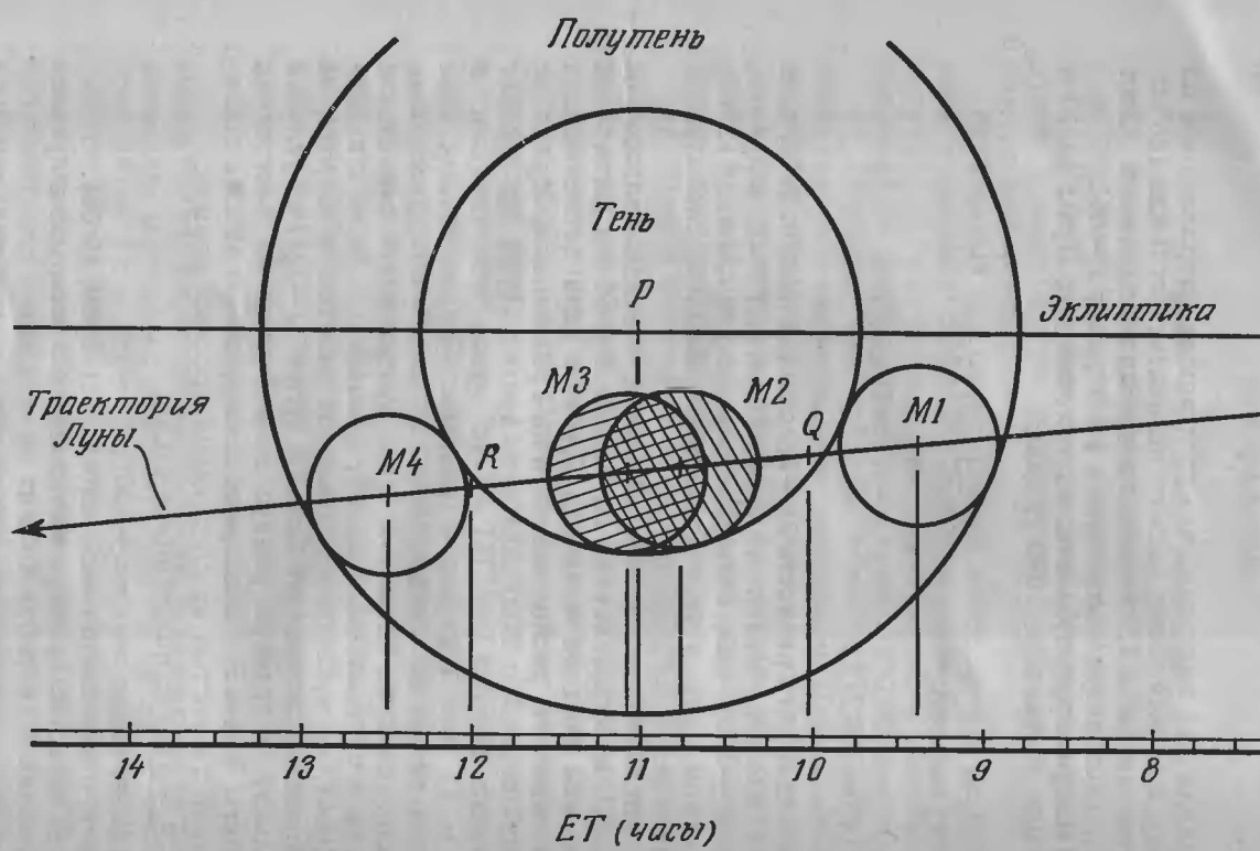
Рис. 39. Лунное затмение 6 сентября 1979 г. Масштаб: 1 ч = 2 см. GMT = ET - 50 с.
