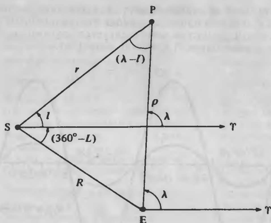
Рис 26 Определение расстояния до планеты
