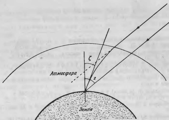
Рис. 12. Атмосферная рефракция.
