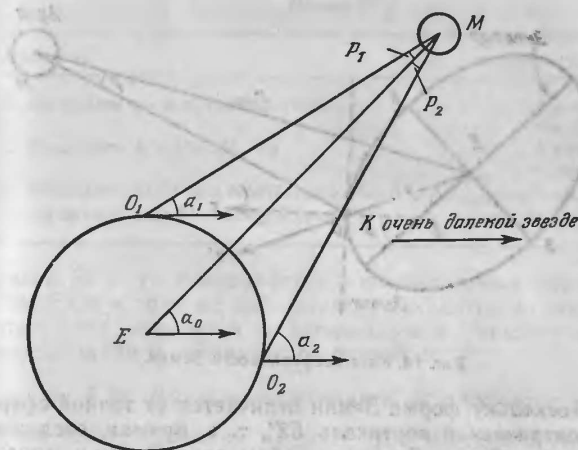
Рис. 13. Геоцентрический параллакс.
