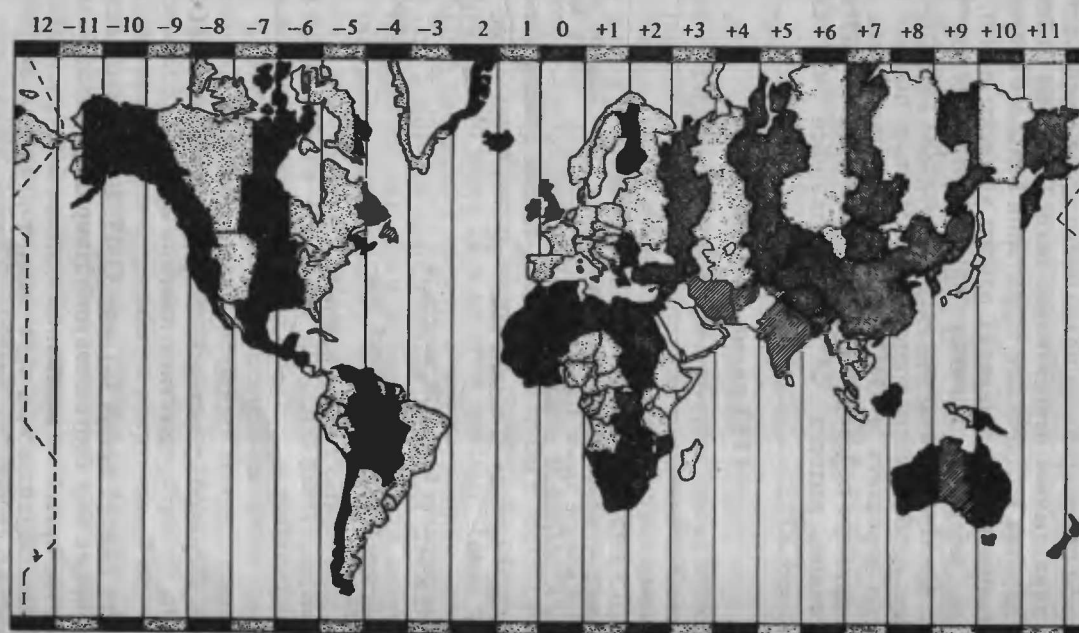
Рис. 2. Карта часовых поясов. На приведенной карте из-за мелкого масштаба видно лишь общее распределение часовых поясов на земном шаре. Если поправка за поясное время неизвестна, то вы можете определить ее по радио сигналам времени, зная поясное время передающей радиостанции
