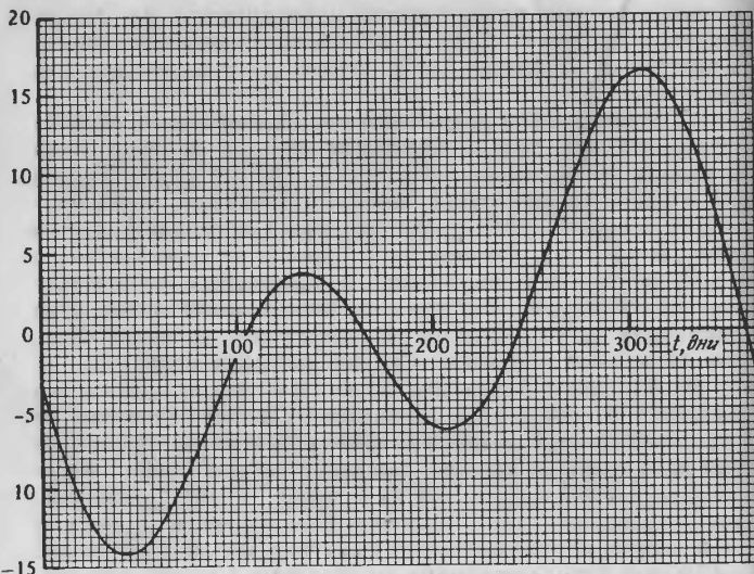
Рис. 20. Уравнение времени.
