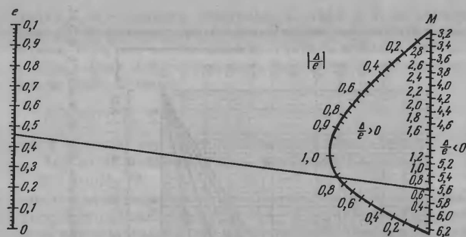
Рис. 29. Номограмма для вычисления \Delta .
