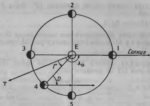
Рис. 35. Фазы Луны.
