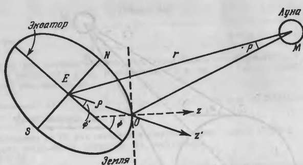
Рис. 14. Учет несферичности Земли.
