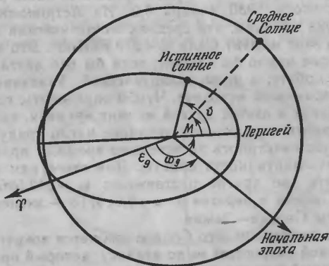
Рис. 18. Определение положения
