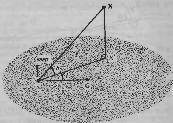
Рис. 8. Галактические координаты.
