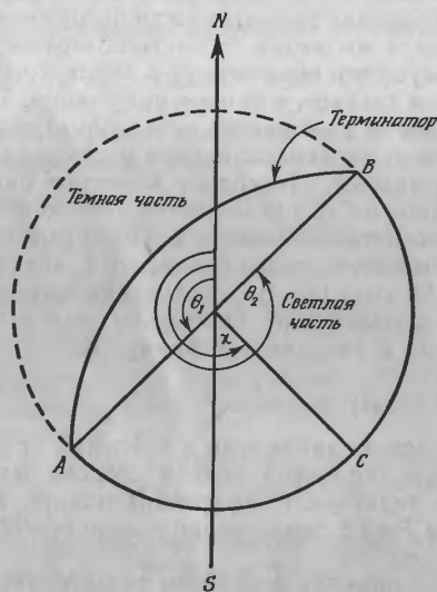
Рис. 27 Позиционный угол светлого лимба.
