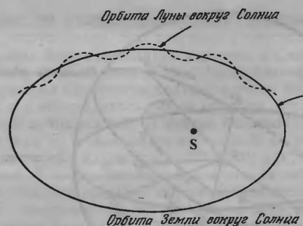
Рис. 32. Лунная орбита (масштаб не соответствует действительности).
