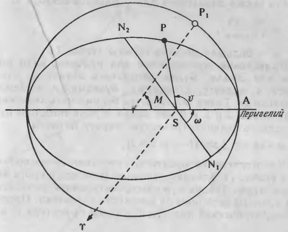
Рис. 22. Средняя и истинная аномалии.
