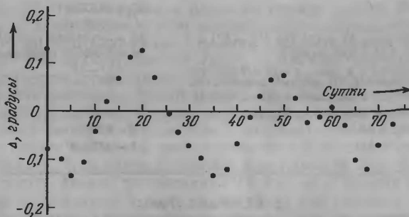
Рис. 34. Разница \Delta = \lambda_m(DS) - \lambda_m(AE) между эклиптическими координатами Луны, вычисленными нашим методом [\lambda_m(DS)] , и приведенными в Астрономическом ежегоднике [\lambda_m(AE)] , для начала 1979 г.
