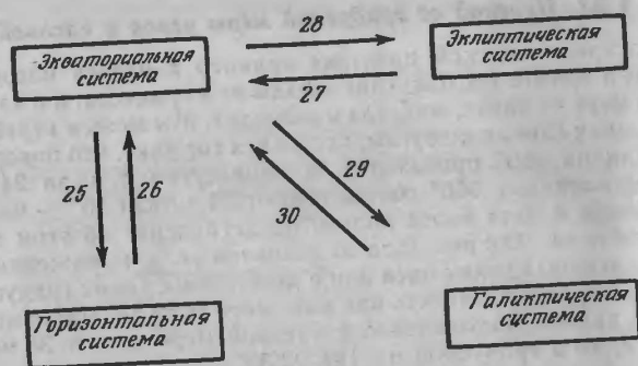
Рис. 9. Переход от одной системы координат к другой.
