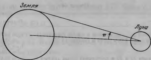
Рис. 36. Параллакс Луны.
