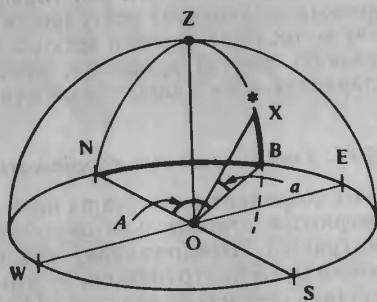
Рис. 5. Горизонтальные координаты.
