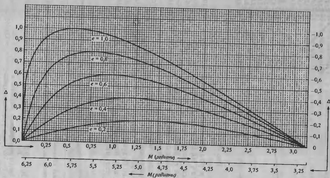
Рис. 28. График уравнения Кеплера. Левая шкала и верхняя шкала M предназначены для M между 0 и 3,14. Правая шкала и нижняя шкала M — для M между 3,14 и 6,28.
