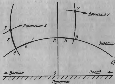
Рис. 6. Экваториальные координаты: а — на небесной сфере; б — при наблюдении с Земли.
