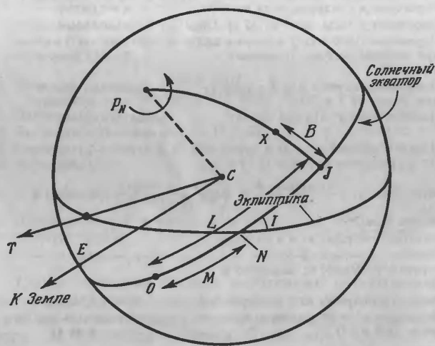
Рис. 15. Определение гелиографических координат
