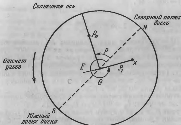
Рис. 16. Солнечный диск.
