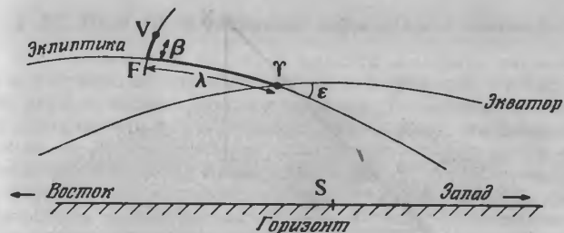
Рис. 7 Эклиптические координаты при наблюдении с Земли
