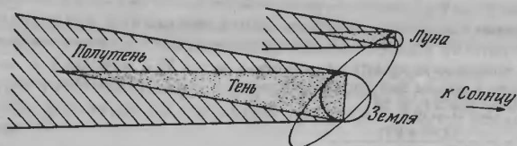
Рис. 37. Тени, отбрасываемые Луной и Землей.
