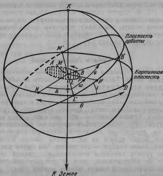
Рис. 31. Орбита двойной звезды.
