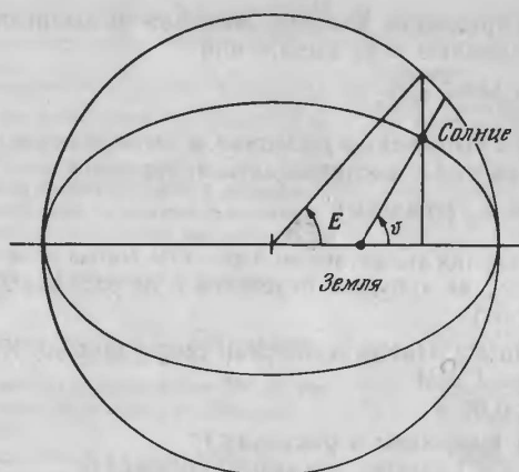
Рис. 19. Истинная аномалия и эксцентрическая аномалия.
