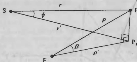
Рис. 24. Определение широты.
