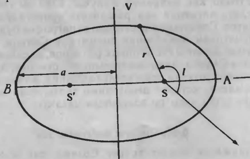
Рис. 17. Эллиптическая орбита.
