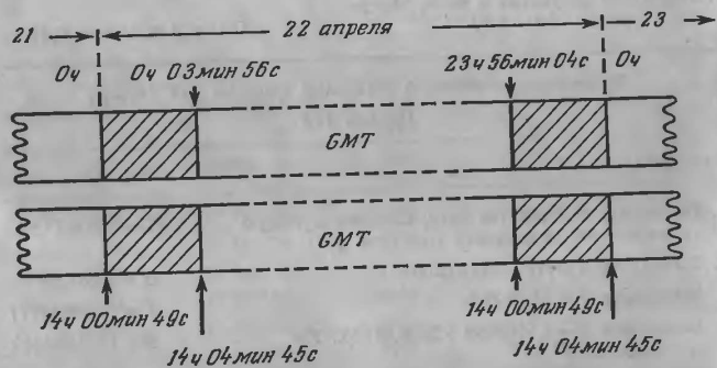
Рис. 3. Соответствие GMT и GST для 22 апреля 1980 г. Заштрихованные интервалы GST повторяются дважды в течение одного и того же дня.
